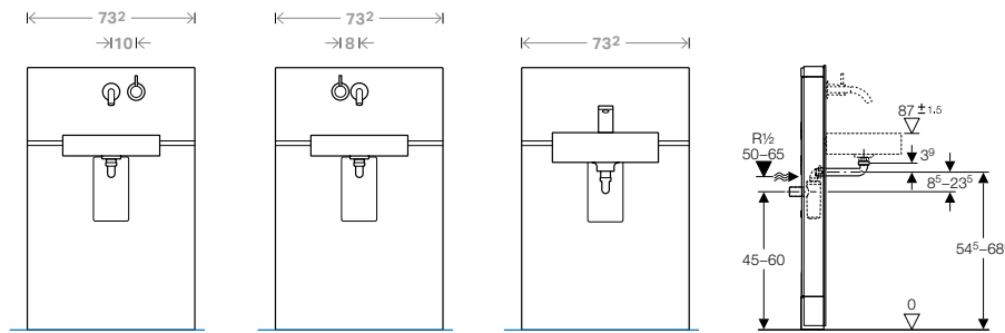
Wandarmatur Hebel rechts für Armaturen mit Stichmass 10 cm
